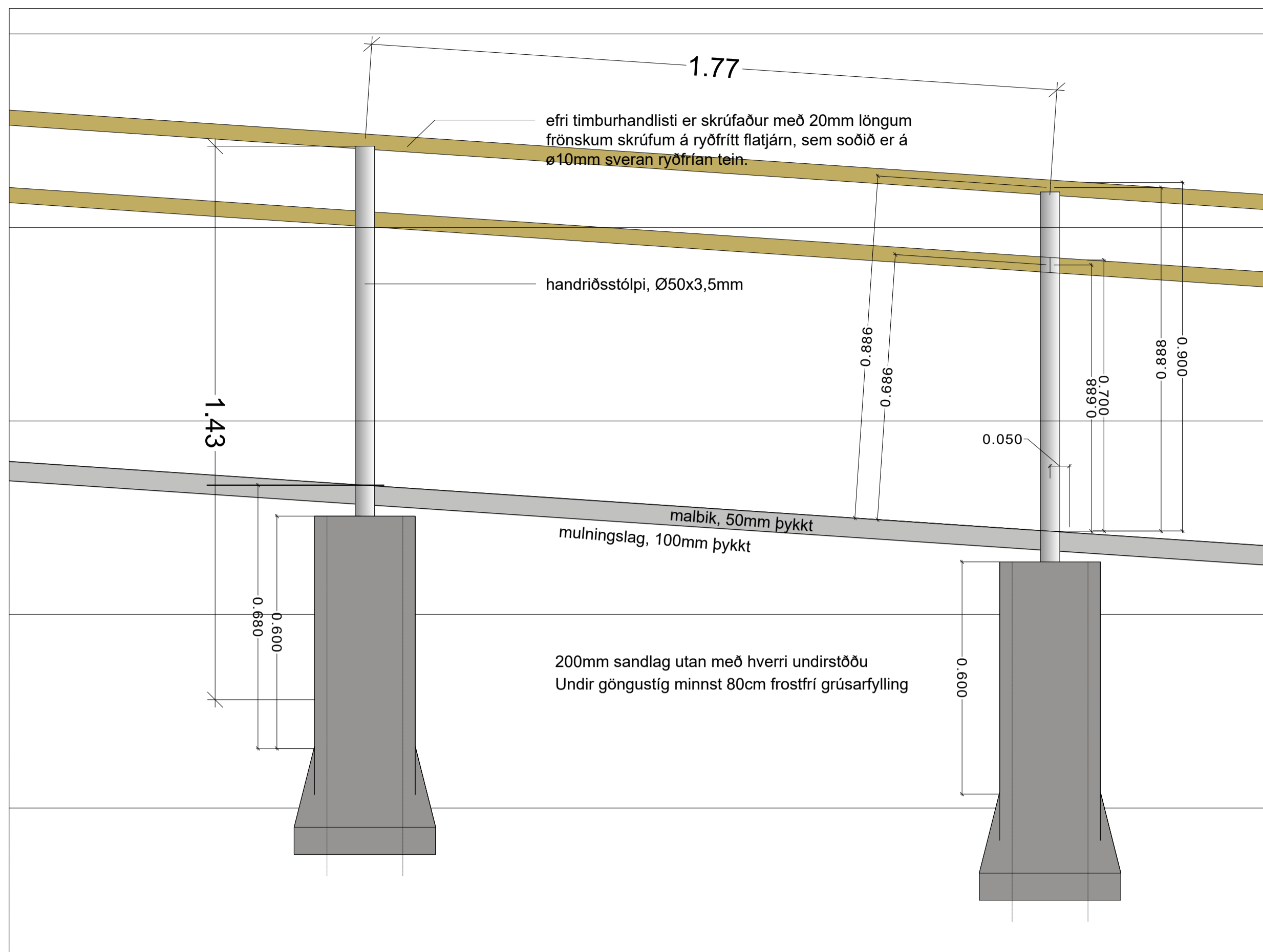
Útlit í handlista við göngustíg - mkv. 1:10
