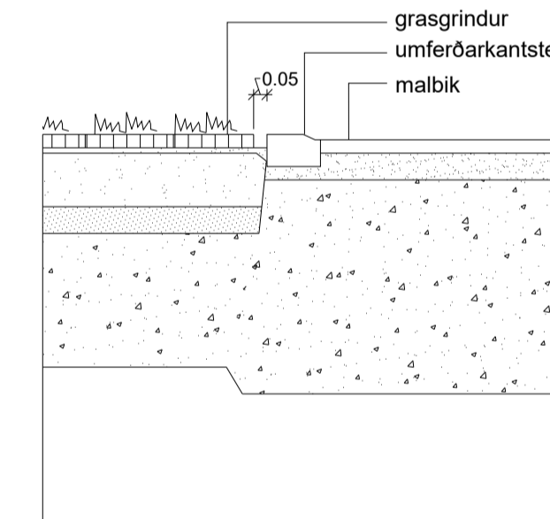
K-1, Umferðarkantsteinn
