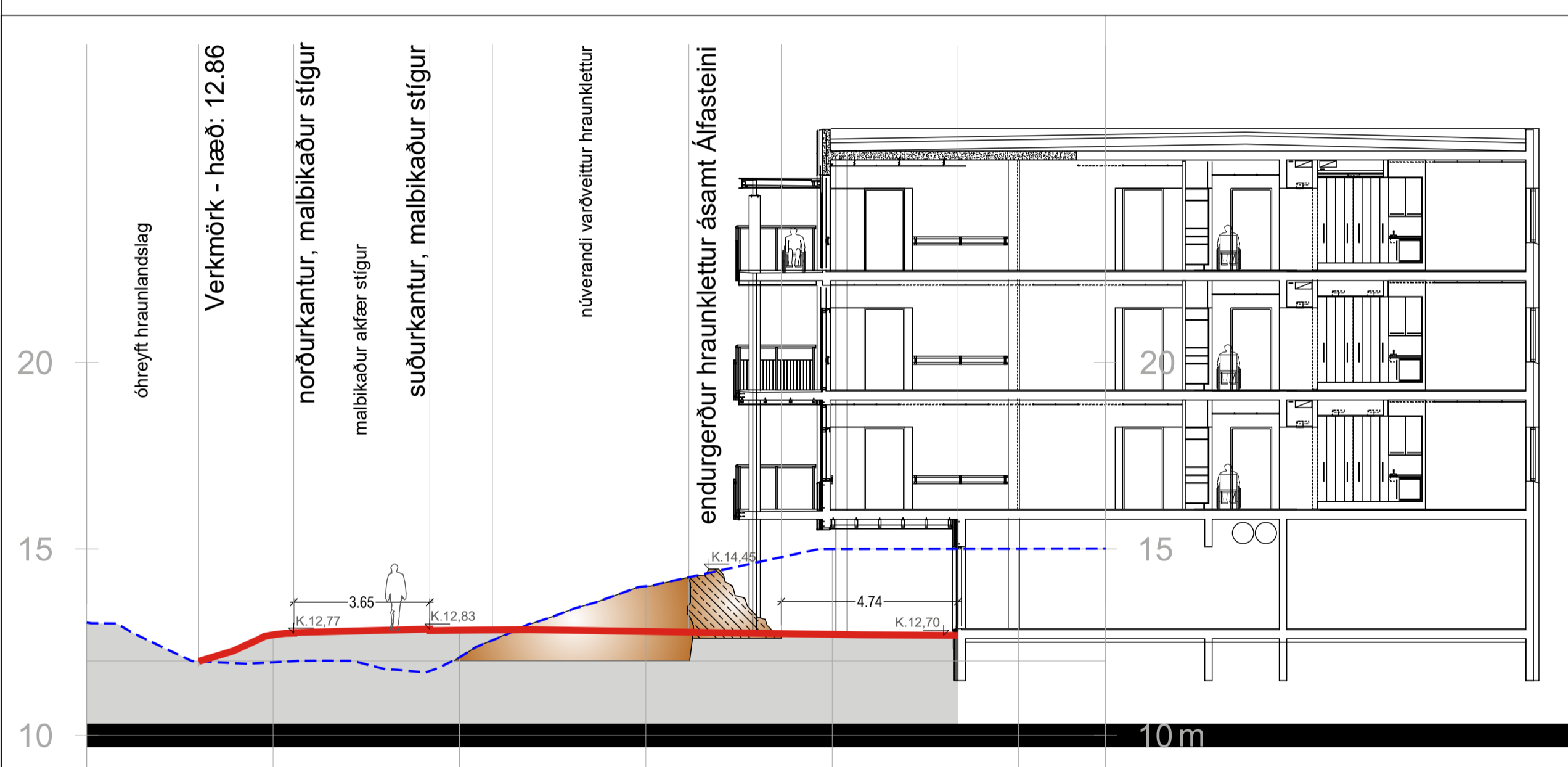
Snið B-B, mkv. 1:125
