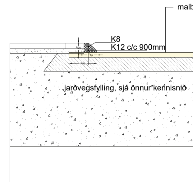
K-4, 10cm vélsteyptur kantsteinn
