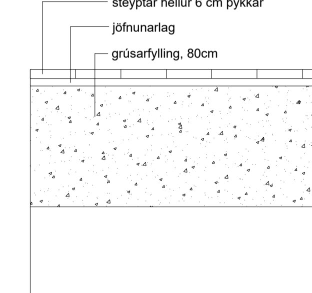
He-1 og He-2 hellur
