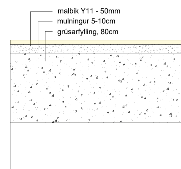
malbik á götur
