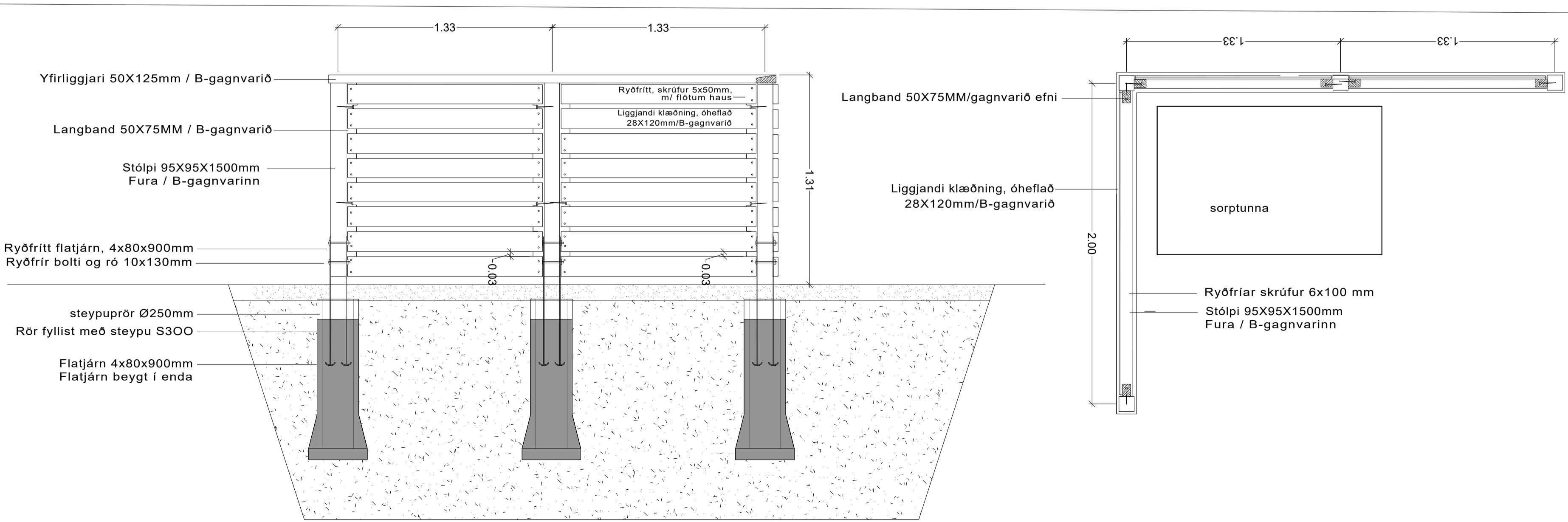
Grunnmynd og útlit í 1,3m háa girðingu við sorpgerði - mkv. 1:20
