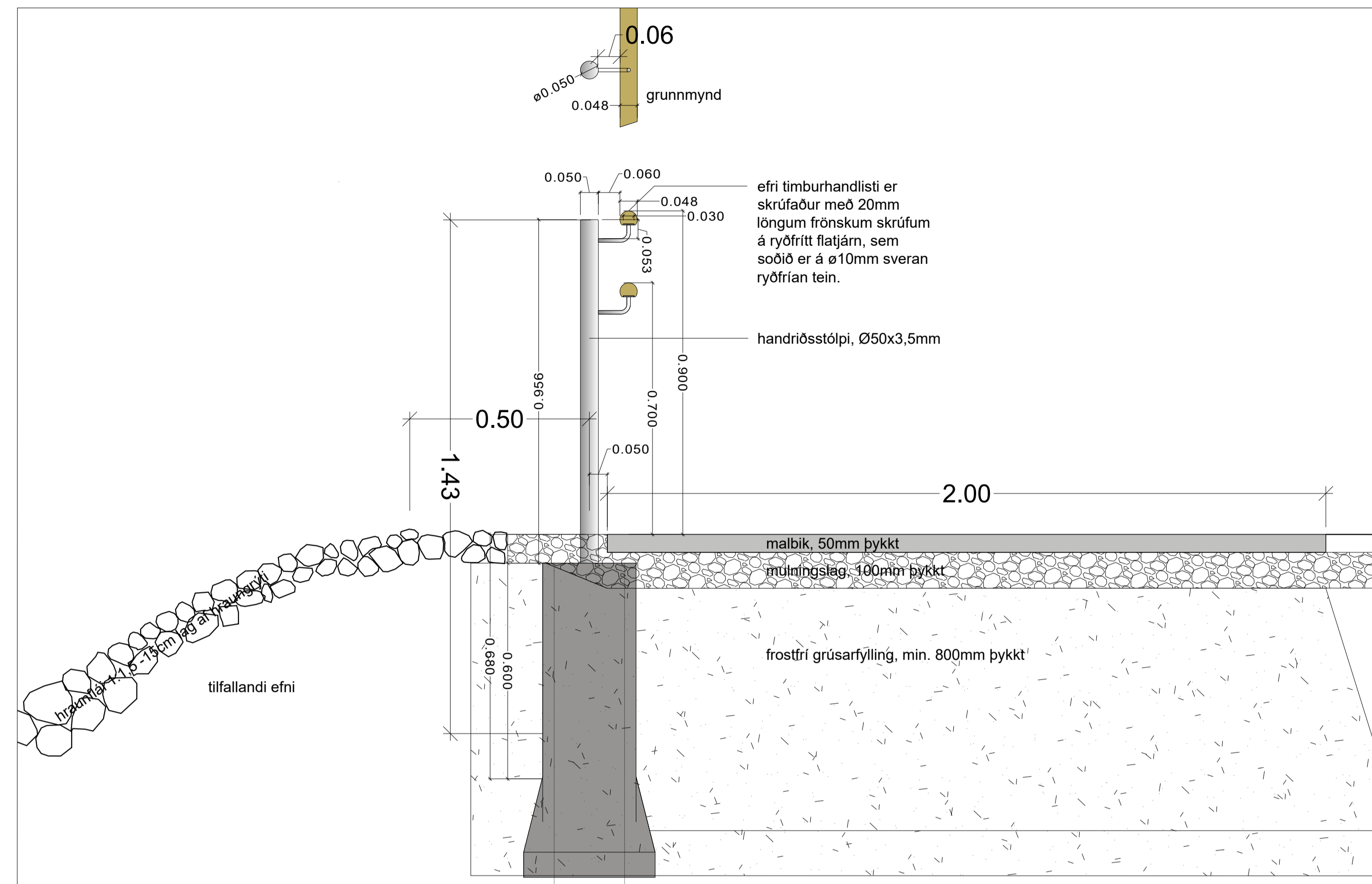
Grunnmynd og þversnið í handlista og göngustíg - mkv. 1:10
