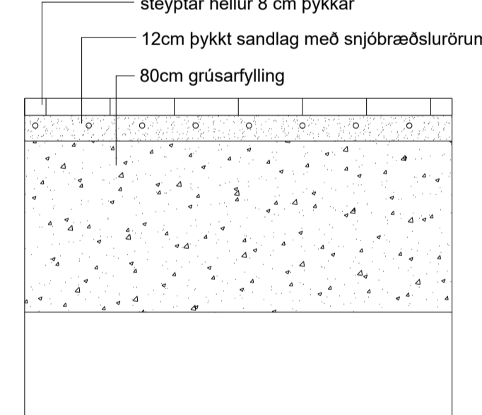
He-4 á snjóbræðslu
