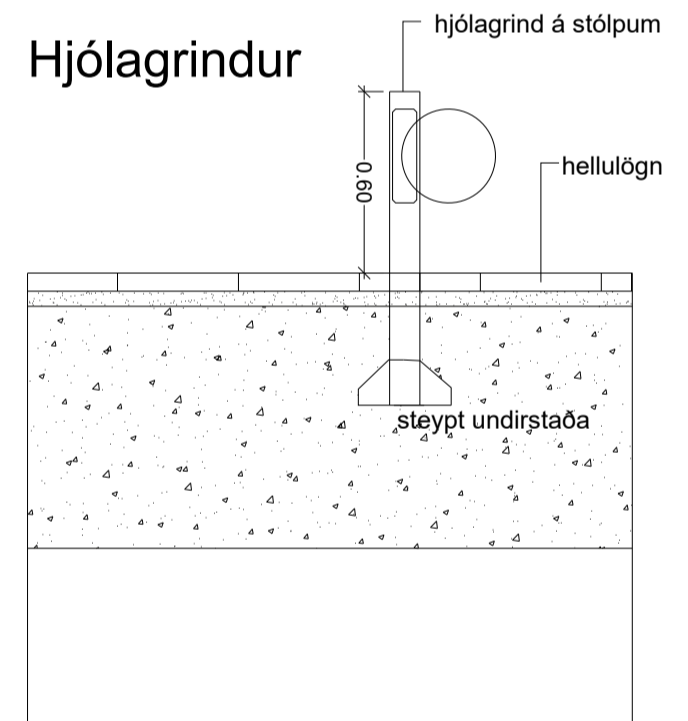
Ýmis kennisnið í frágang - mkv. 1:25
