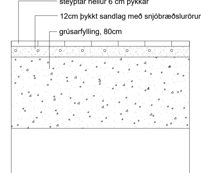
He-1 og He-2 á snjóbræðslu
